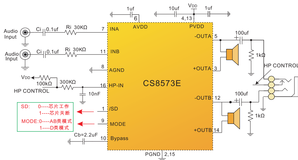
图 1 CS8573E应用线路图
