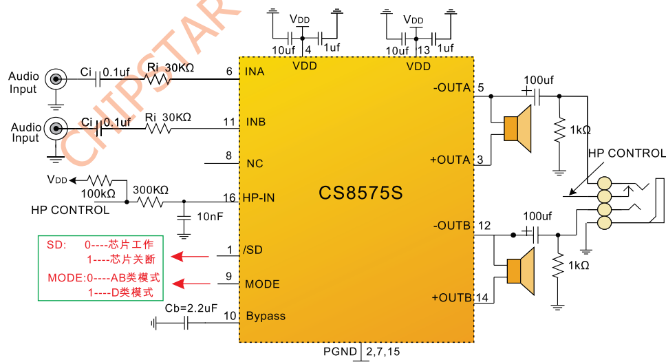
图 1 CS8575S应用线路图
