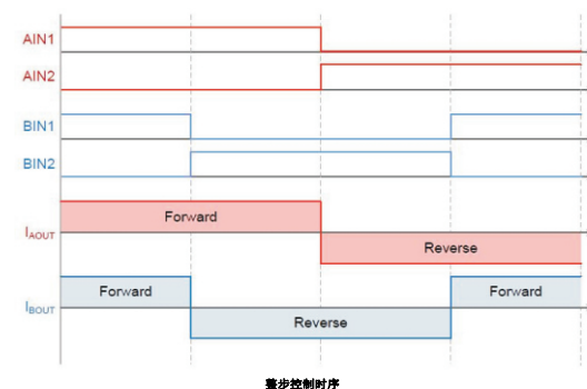
整步控制时序
