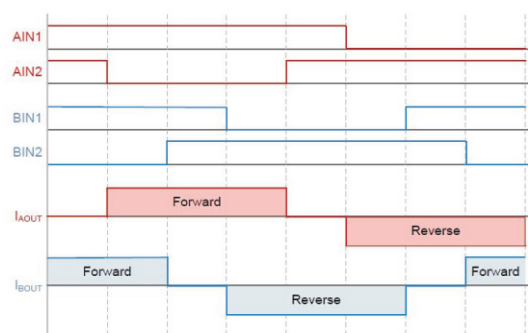
半步控制时序
