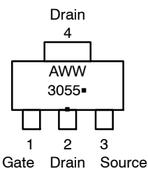
SOT-223 CASE 318E STYLE 3
