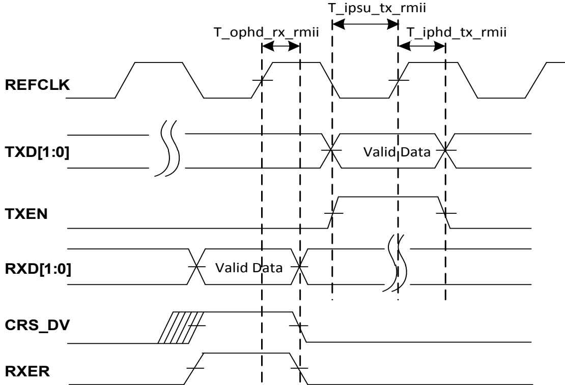
图 27.RMIi 传输和接收周期时序
