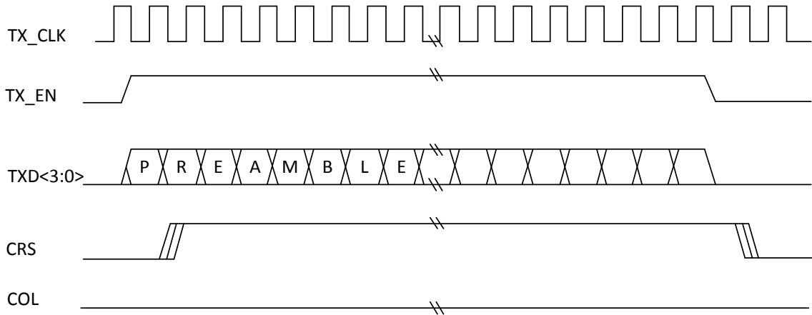
图 30.MAC 到 PHY 无冲突的发送
