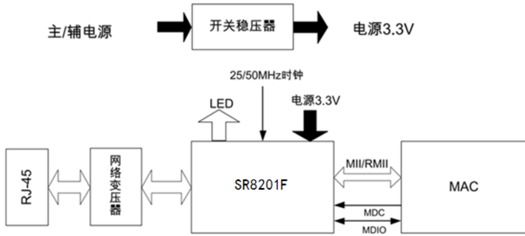
图 2. 应用框图
