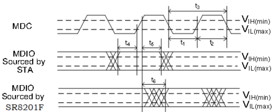
图 29.MDC/MDIO时序
