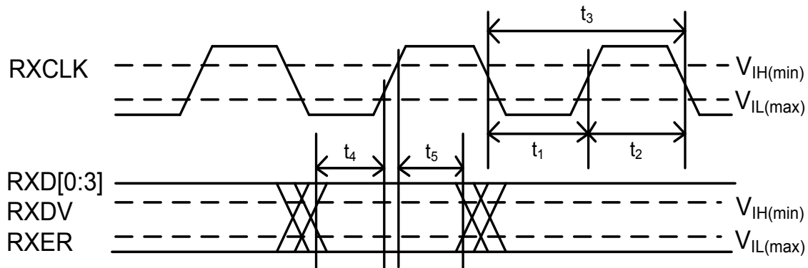
图 24.MII 接收周期时序-1
