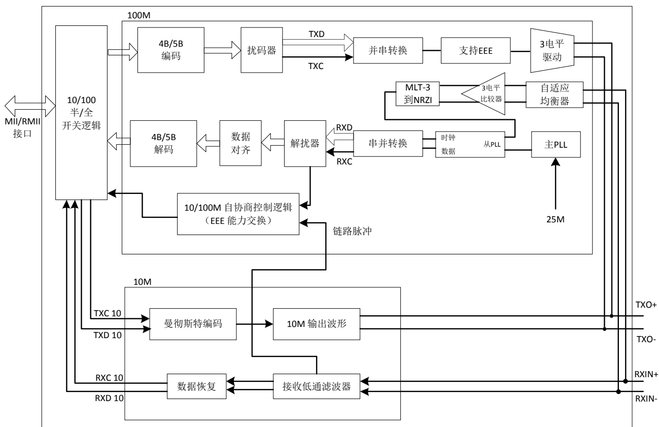
图 1. 内部框图
