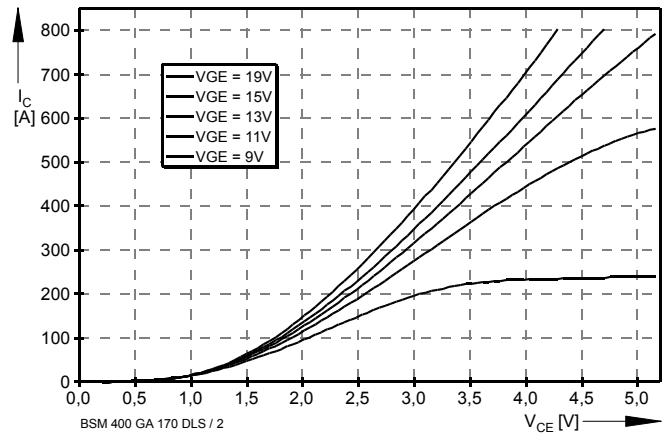
Bild / Fig. 2 Ausgangskennlinienfeld (typisch) / Output characteristic (typical) I_C = f(V_{CE}) T_{Jj} = 125^\circ C
