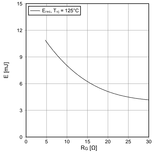
Schaltverluste Diode-Wechselr. (typisch) switching losses diode-inverter (typical) E_{rec} = f(R_G) I_F = 200 A, V_{CE} = 600 V
