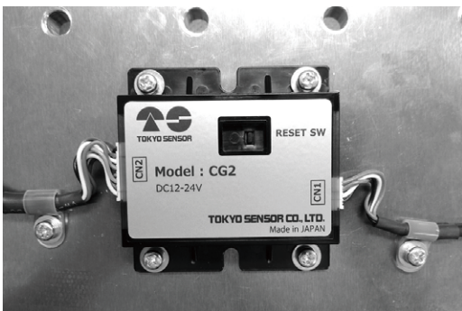
主体安装例
