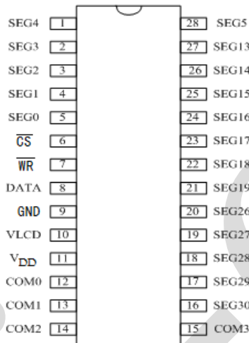
SOP28
