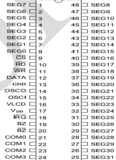
SSOP48
