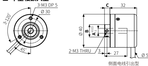
侧面电线引出型
