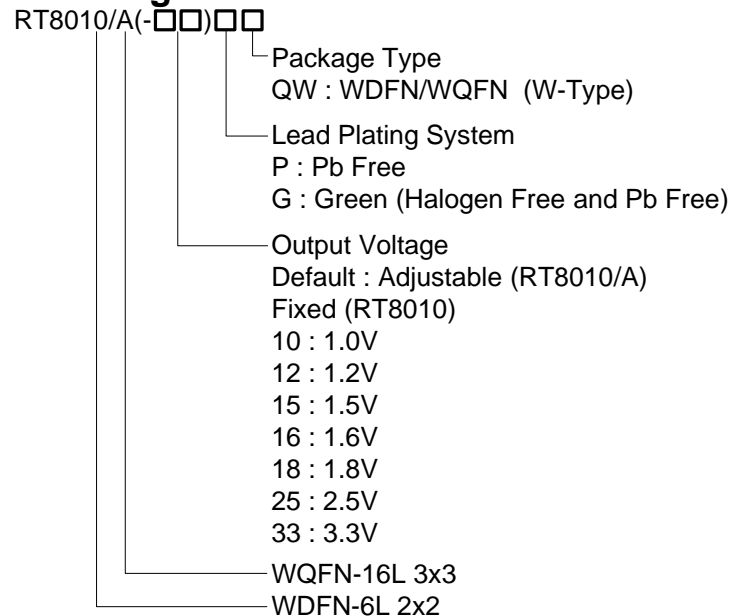
WQFN-16L 3x3 (RT8010A)
