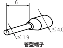
管型端子
