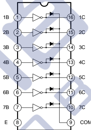
图 2 ULN2004管脚定义图
