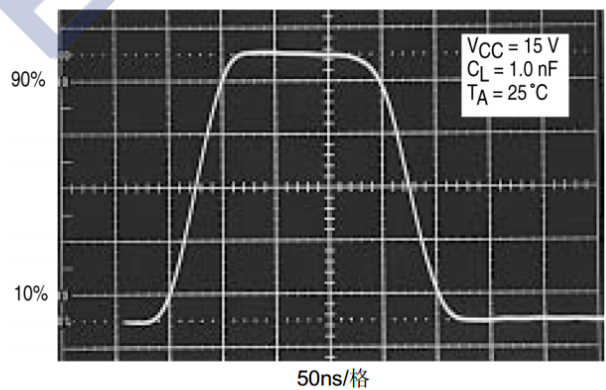
图 12. 输出波形
