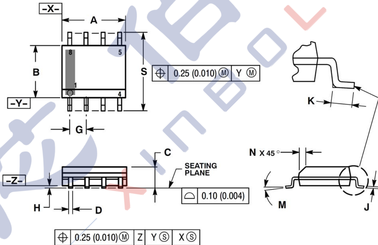
8 引脚塑料 SOP
