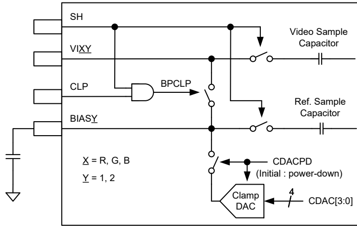
图 1 偏压和钳位配置
