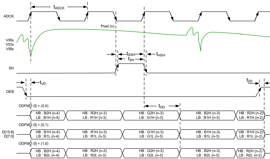
图 3 S/H 及数据输出控制时序
