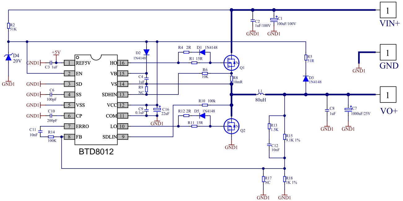
图 6-1. BTD8012 12V10A 典型应用电路图
