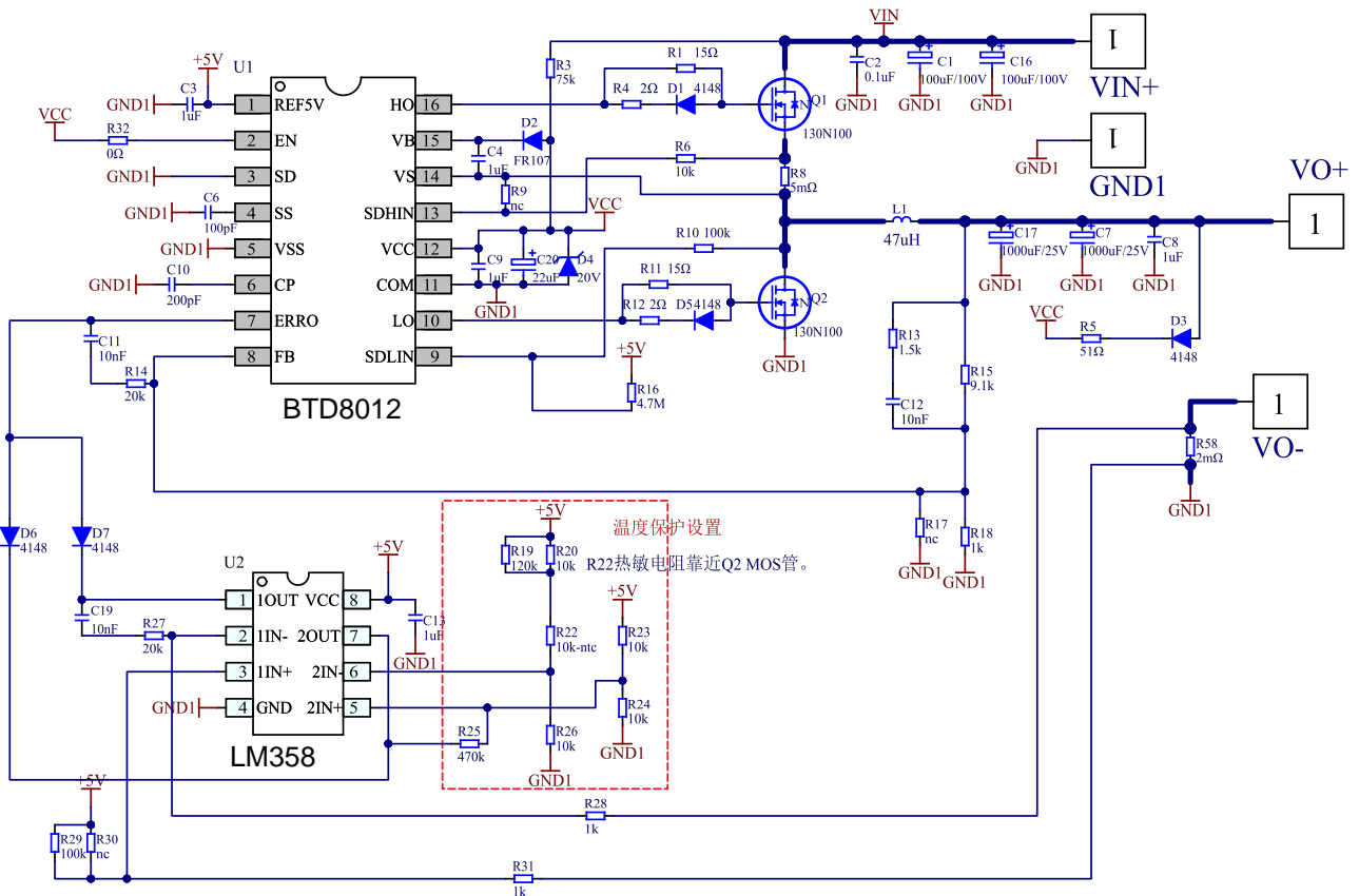
图 6-2. BTD8012 12V 20A 电恒压恒流同步整流方案典型应用电路图
