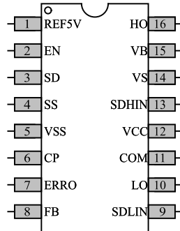
图 4-1. BTD8012 管脚定义
