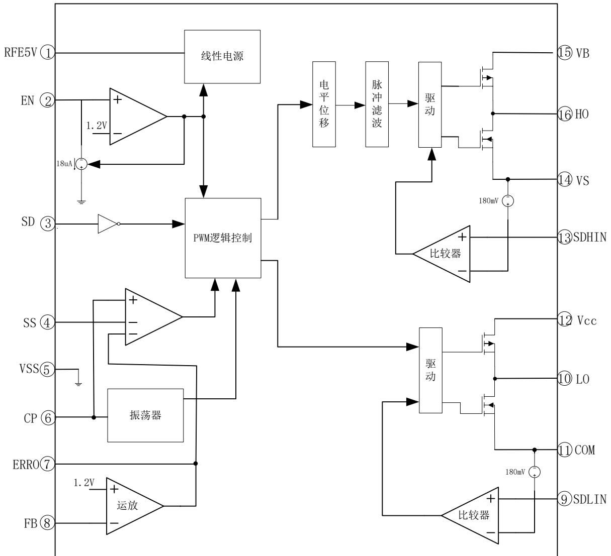
图 5-1. BTD8012 结构框图
