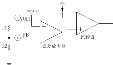
图 8.10a BTD8012 输出电压调整电路
