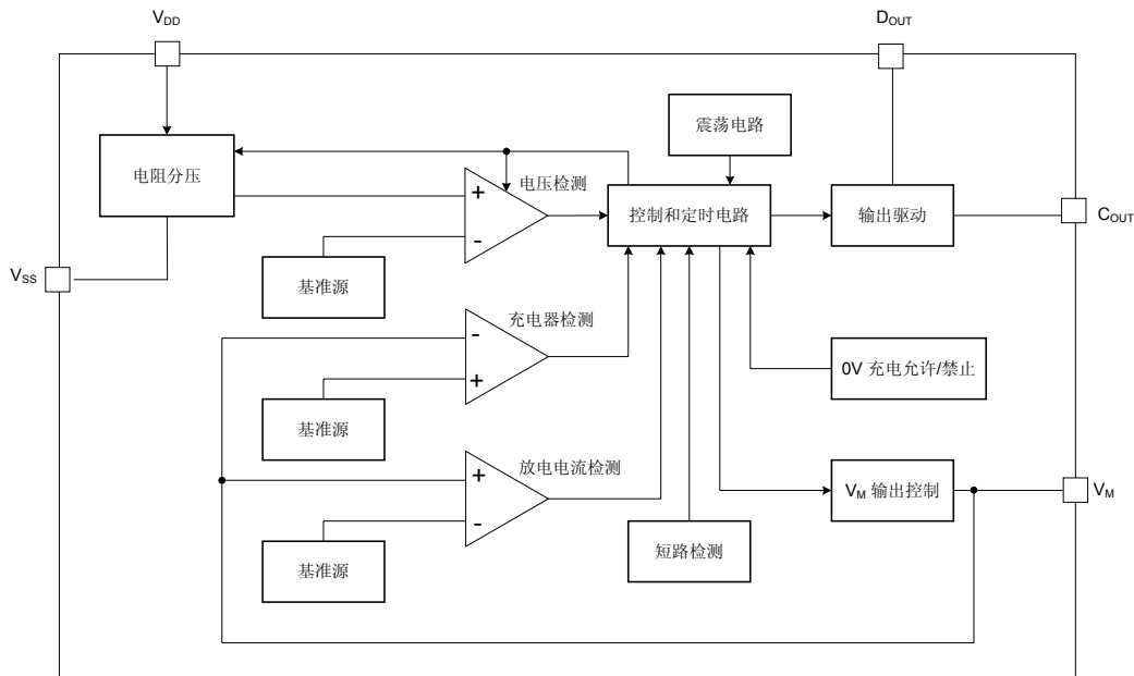
图-3 PL7071 功能框图
