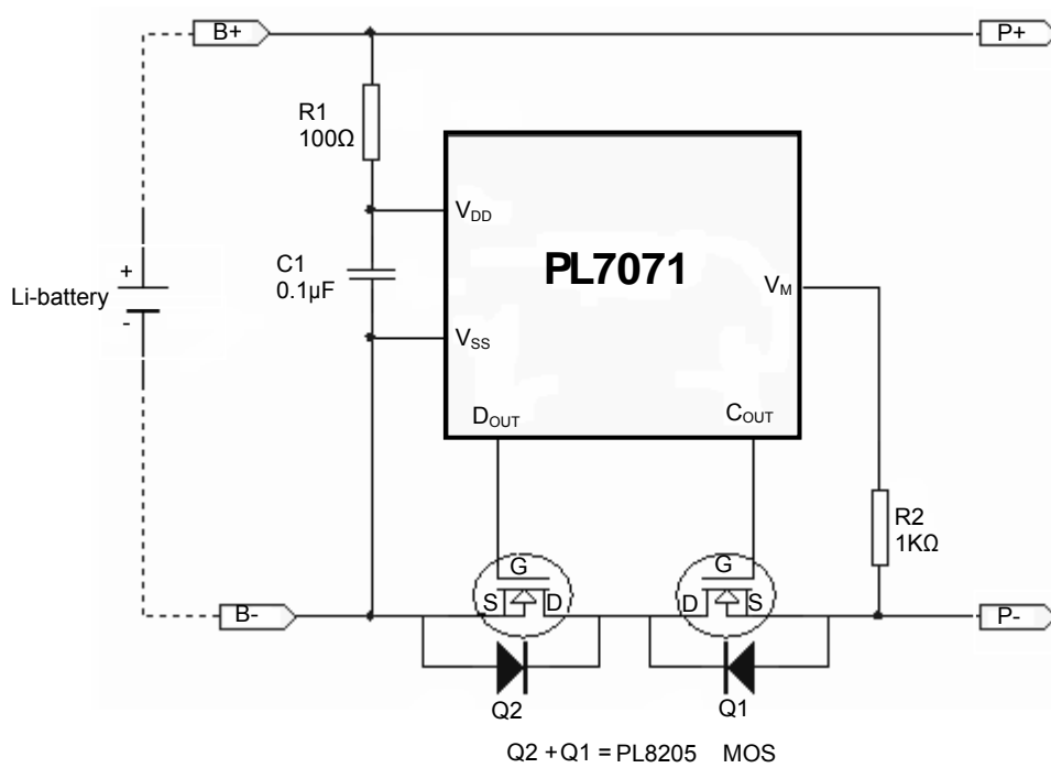
图-2 PL7071 典型应用电路图
