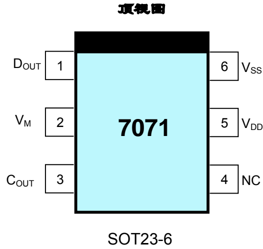
图-1 PL7071 管脚排列 (不成比例)
