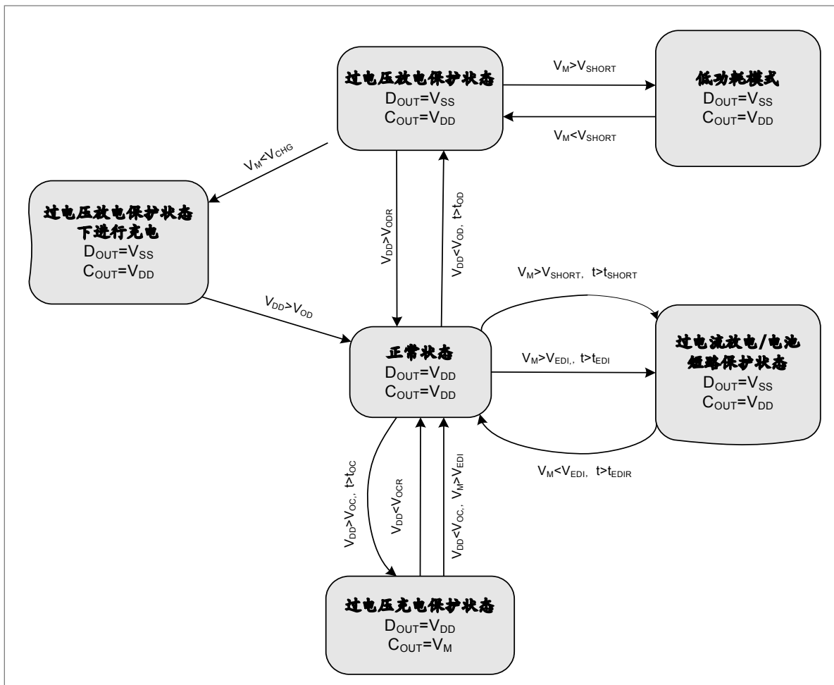
图-4 PL7071 各状态之间的转换图
