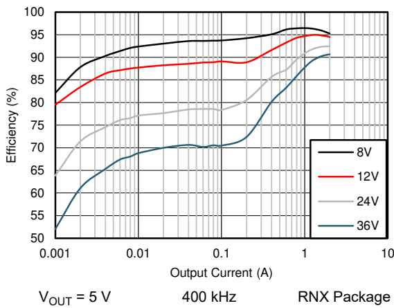
图 8-11. Efficiency
