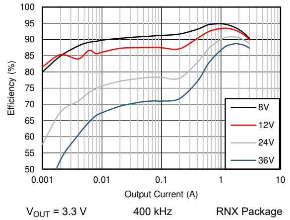
图 8-10. Efficiency
