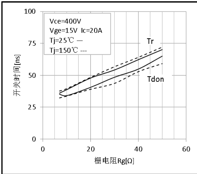
图 5 开通时间与栅极电阻的关系 (感性负载，测试电路参考图 E)
