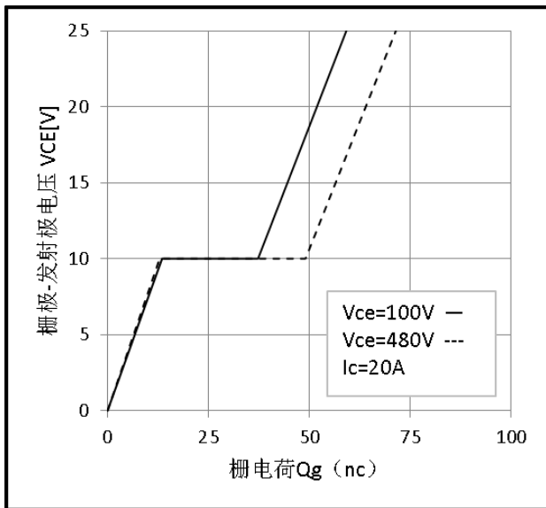
图 15 栅电荷特性
