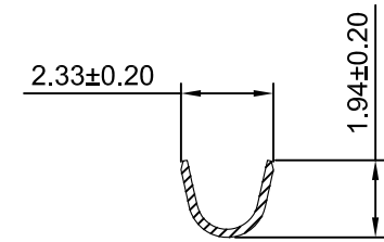
SEC:A-A
