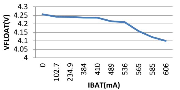
浮充电压与充电电流关系
