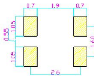
建议焊盘尺寸
