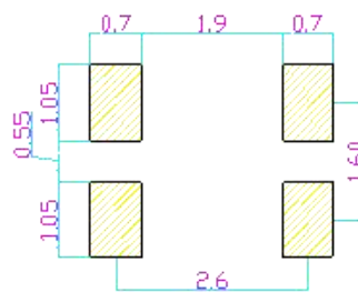
建议焊盘尺寸
