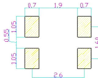
建议焊盘尺寸
