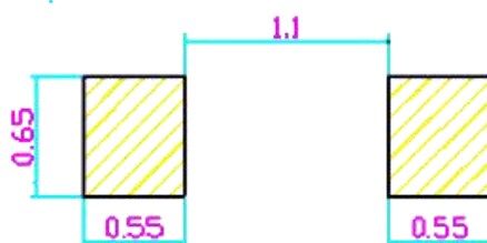
推荐焊盘尺寸
