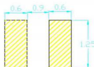
建议焊盘尺寸
