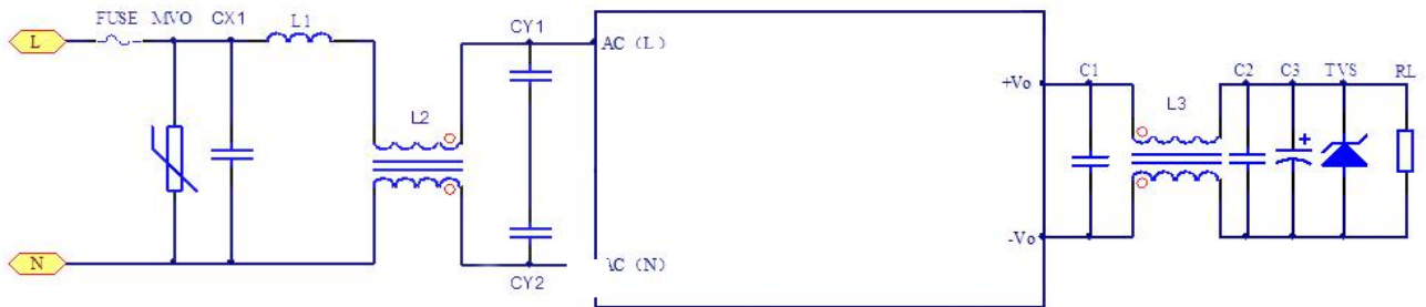
(图 1: EMC 推荐电路)
