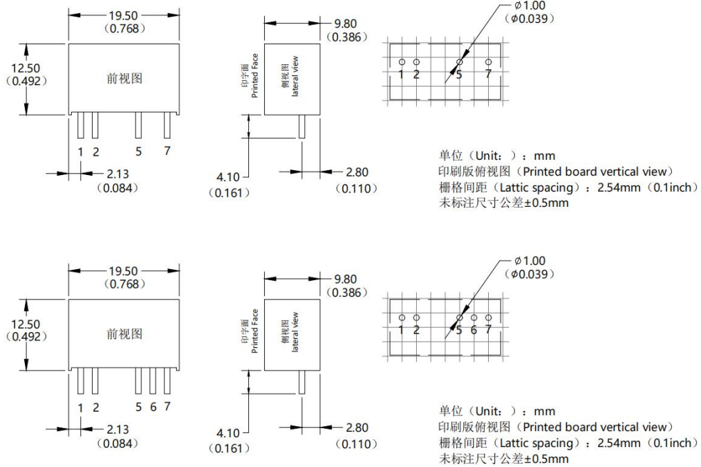
封装尺寸图
