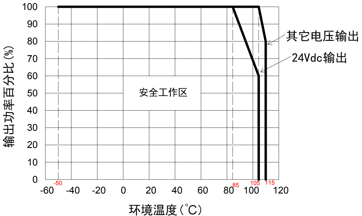
温度降额曲线图
