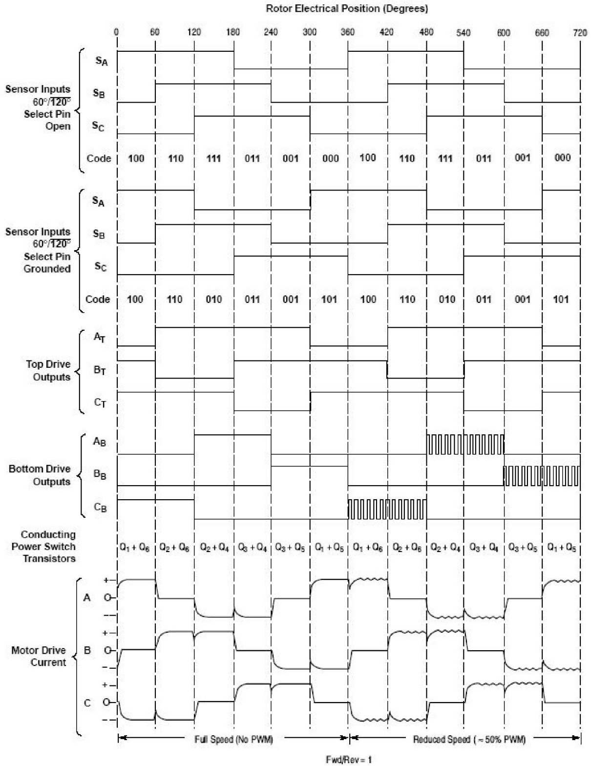
图 37. 三相、六步、全波换向波形
