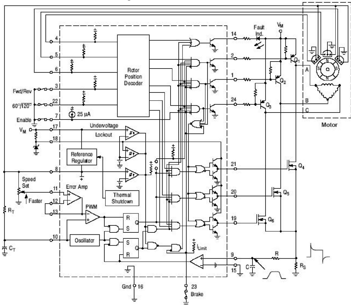
图 36. 三相、六步、全波电机控制电
