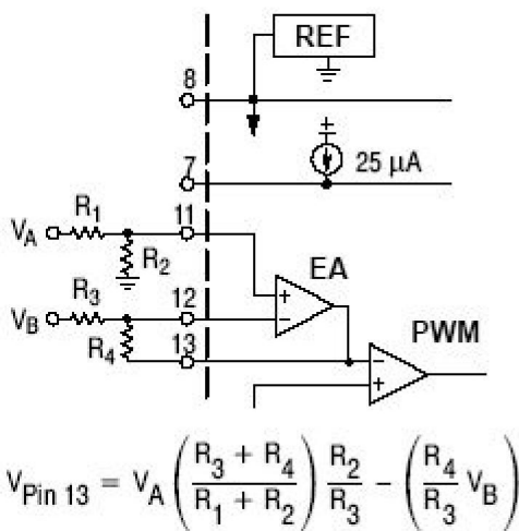
图 31. 速度控制的差分输入器
