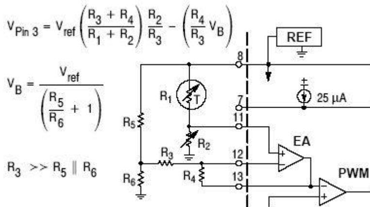
图 35. 闭环温度控制
