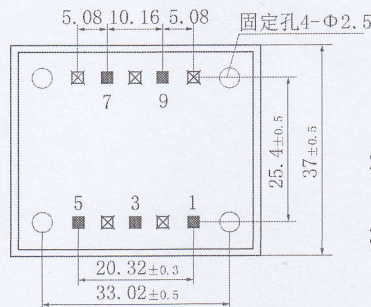
注：■ 有针脚，□ 无针脚 底视图（做PCB板时需注意）
