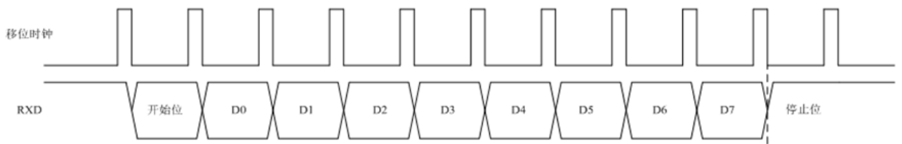
图 2-2 UART 接收数据波形
