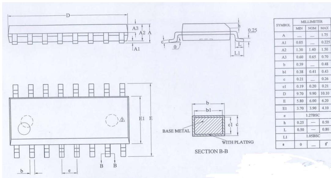
图 7-1 CS1270 SOP16 封装外形尺寸说明
