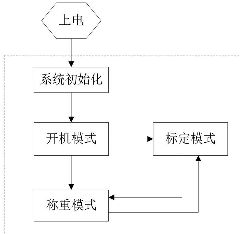
图 3-1 工作模式图
