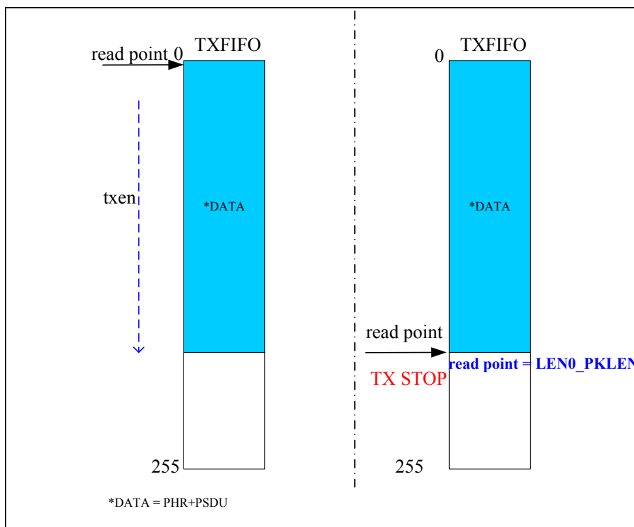
图 8-4 直接 FIFO 帧结构 LEN0_TXMODE='0'发送停止示意图
