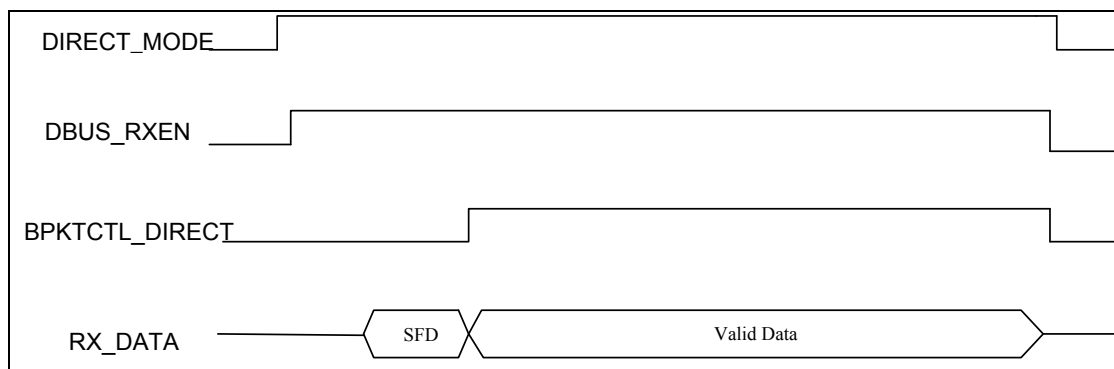
图 8-7 直接接收模式时序图
