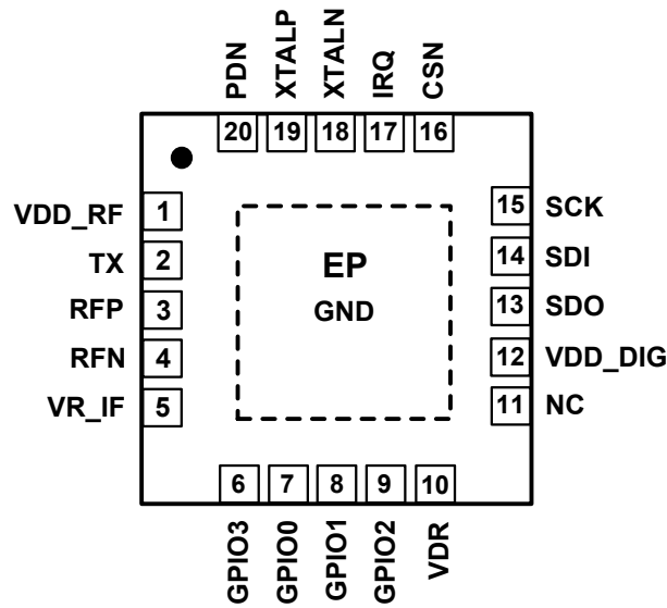
图 1-2 HW3000 QFN20 封装示意图
