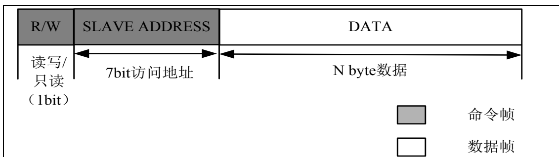
图 6-14 SPI 帧格式
