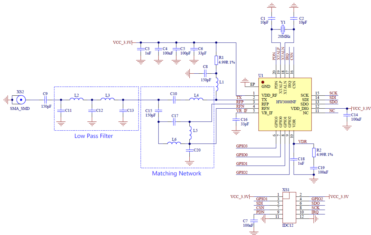
图 13-1 HW3000 Direct Tie 结构典型应用原理图
