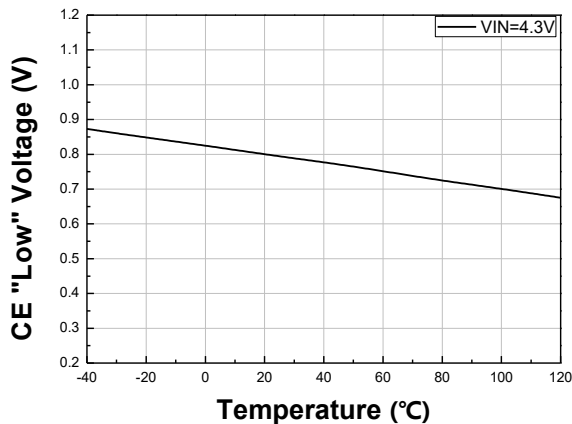
11. CE最大低电平 VS 温度
