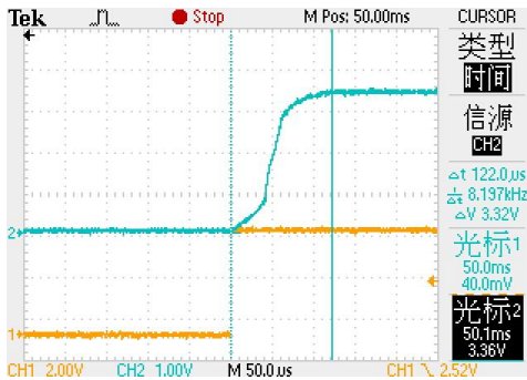
17. CE启动时间
