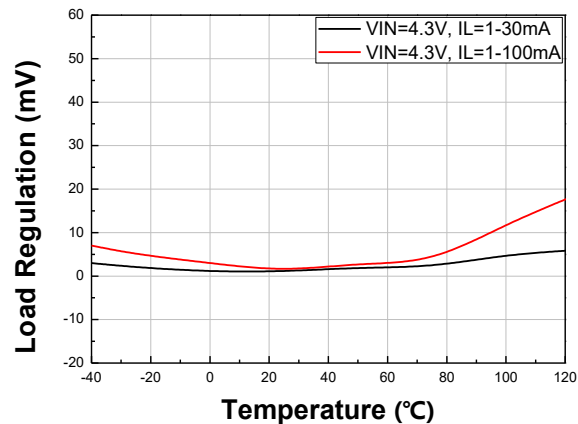
12. 负载调整度 VS 温度
