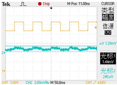
15. 负载瞬态响应(IL=10-350-10mA)
