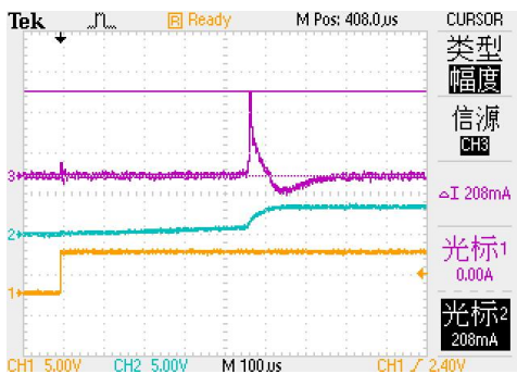
19. 浪涌电流 (IRUSH)
