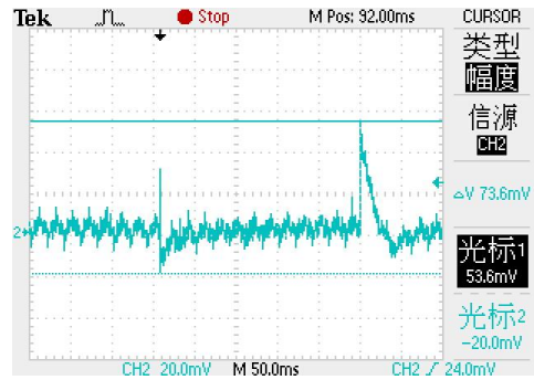
16. 纹波抑制比 (IL=50mA, Vpp=1V, F=1KHZ)
