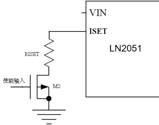
图 5. LN2051的使能设计
