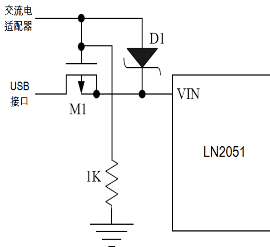
图 4. 同时使用交流电适配器和 USB 接口
