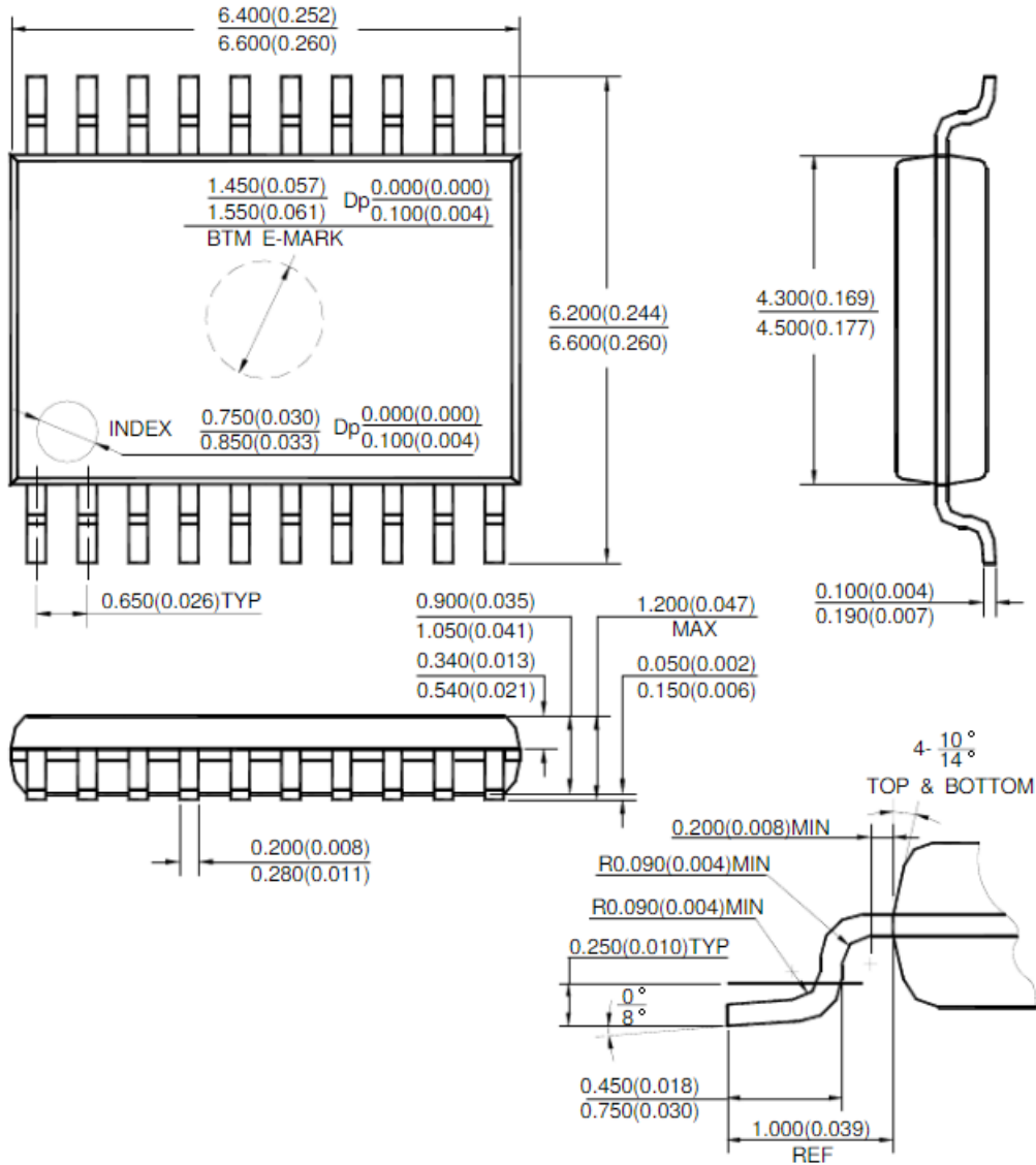
TSSOP-20
