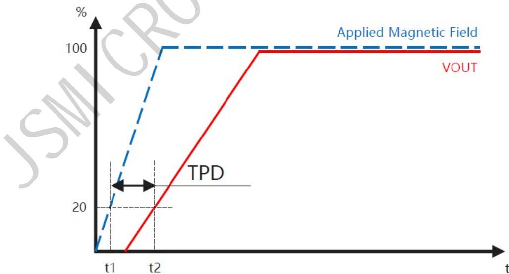
图 2: 传输延迟定义
