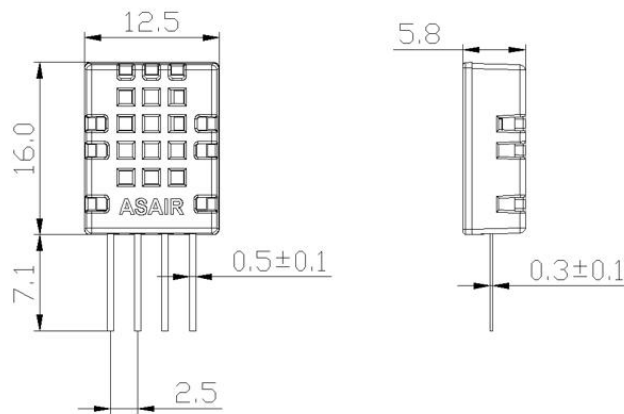
图5. AGS02MA尺寸图，未注公差±0.5mm（单位：mm）
