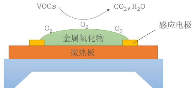
图 2. AGS02MA 原理示意图
