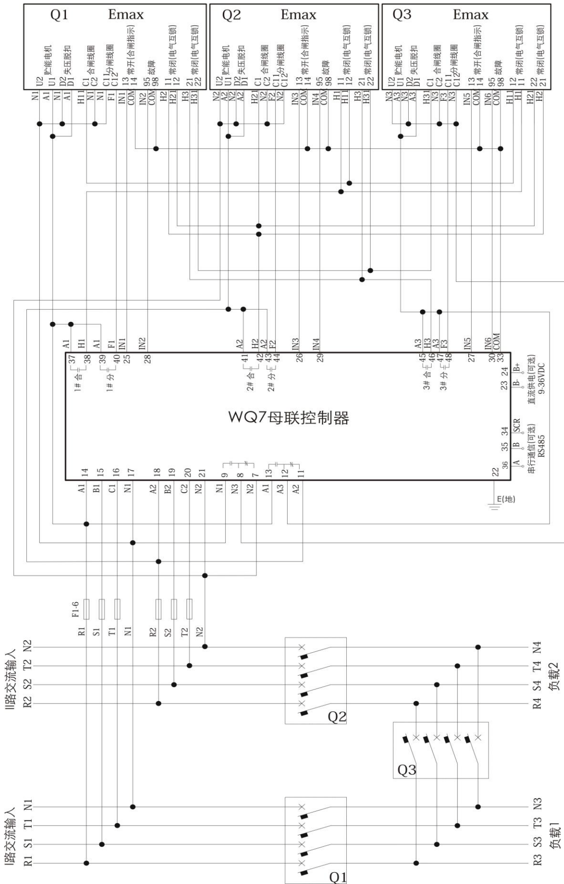
WQ7C 用于 Emax 接线图
