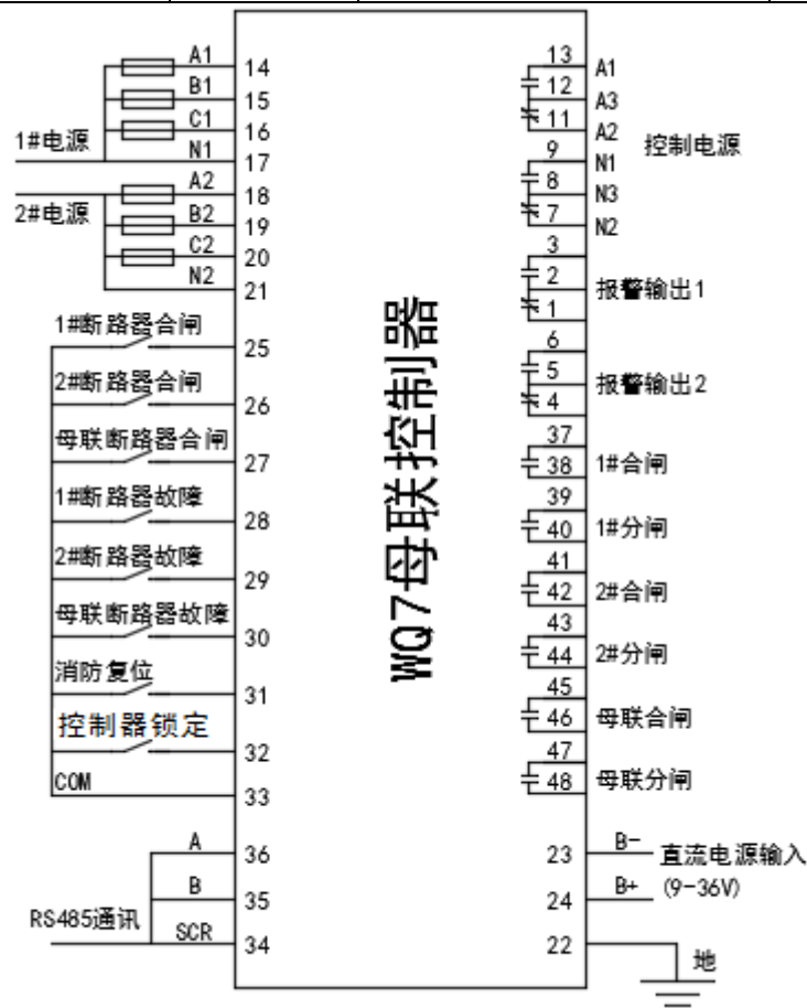
应用原理图
