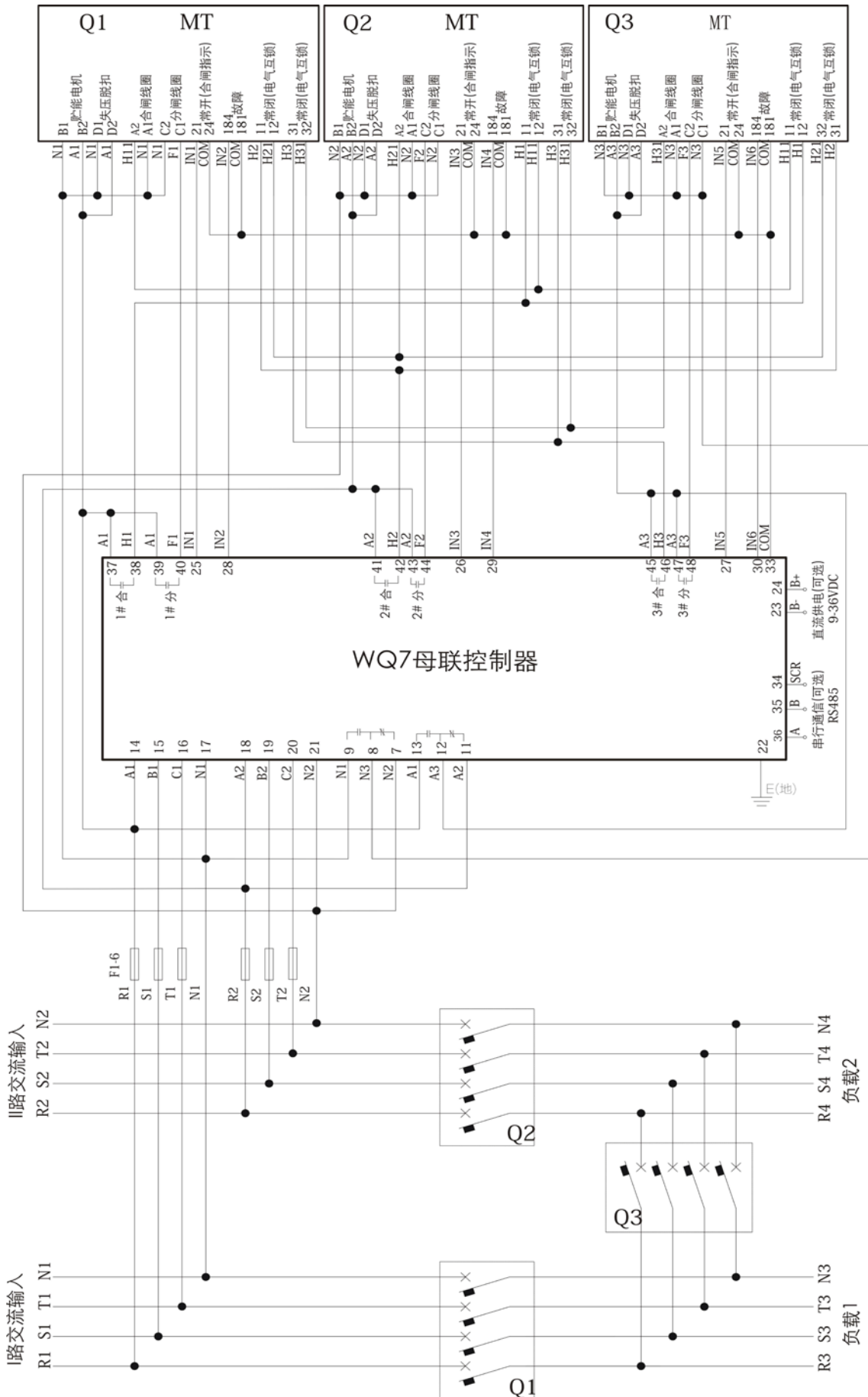
WQ7C 用于施耐德 MT 接线图
