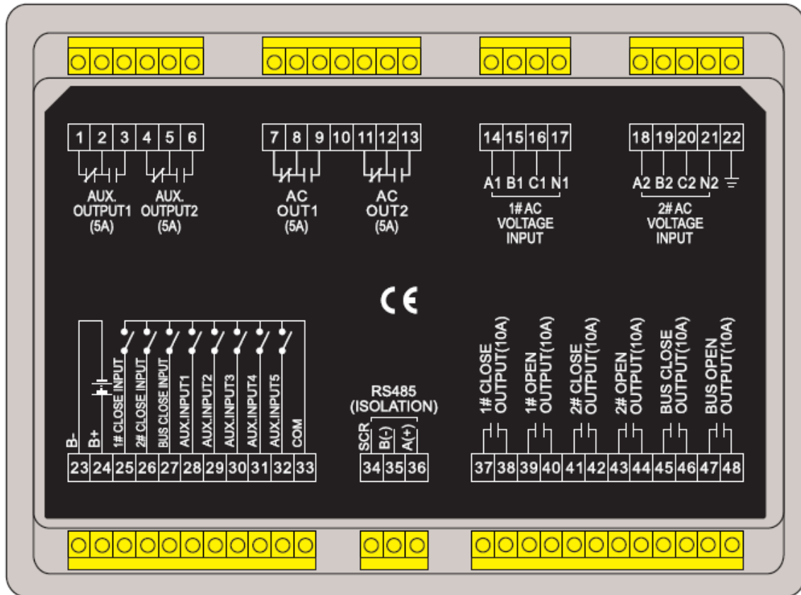
控制器后面板图
