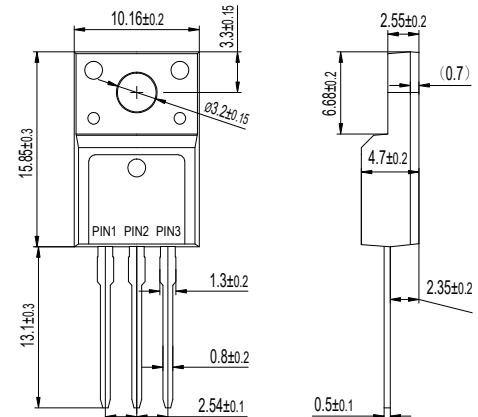
ITO-220AB
