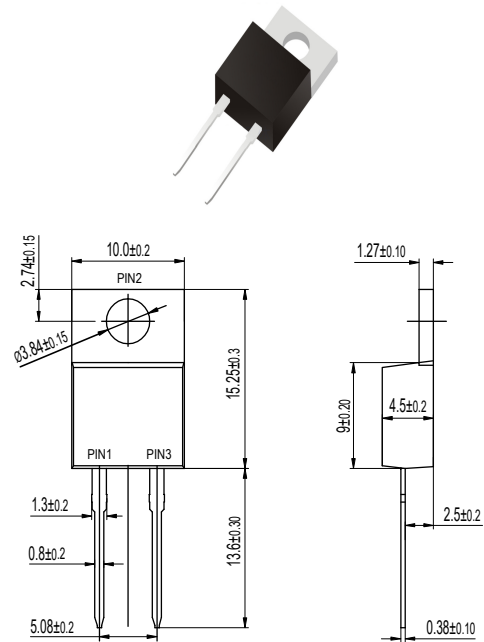
TO-220AC
