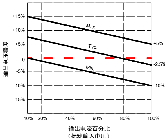
其它电压输出 误差包络曲线图
