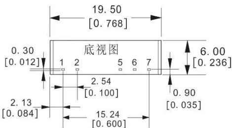
封装尺寸图
