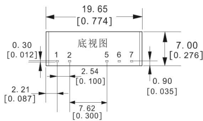
封装尺寸图
