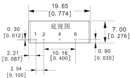
封装尺寸图
