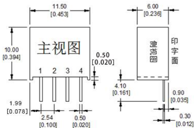
封装尺寸图
