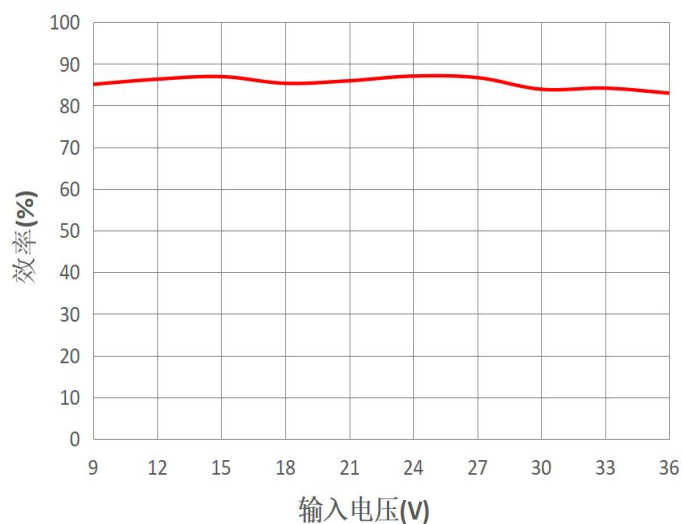
效率 VS 输入电压 (PFD6-36S12A3(C)2)
