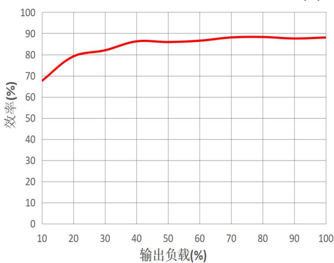
效率 VS 输出负载 (PFD6-36S12A3(C)2)
