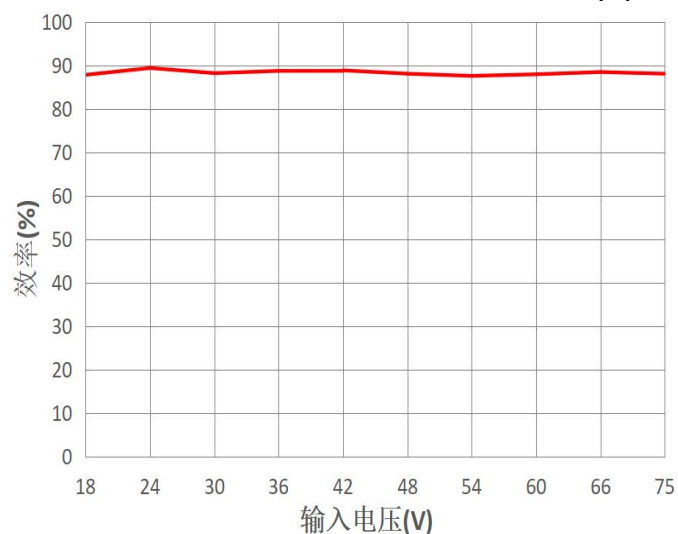
效率 VS 输入电压 (PFD6-36S12A3(C)2)
