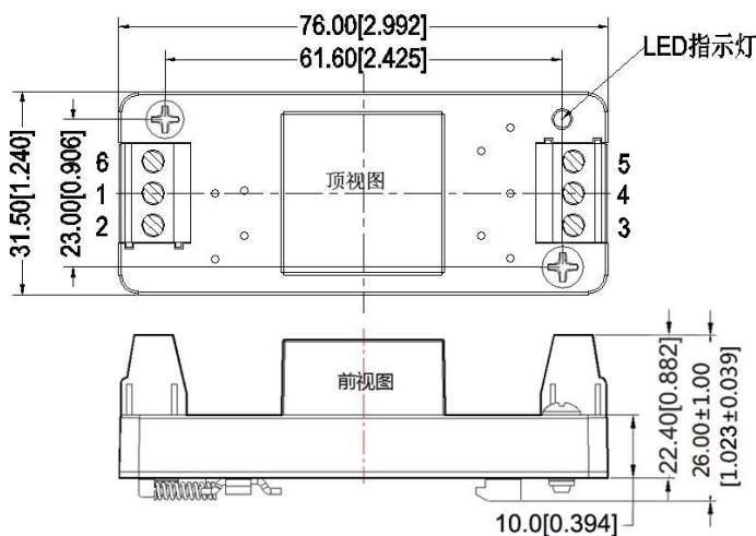
引脚定义
