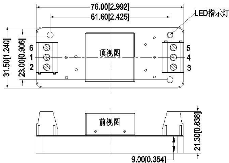
引脚定义
