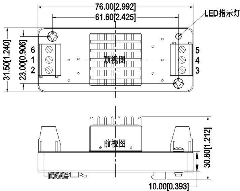
引脚定义
