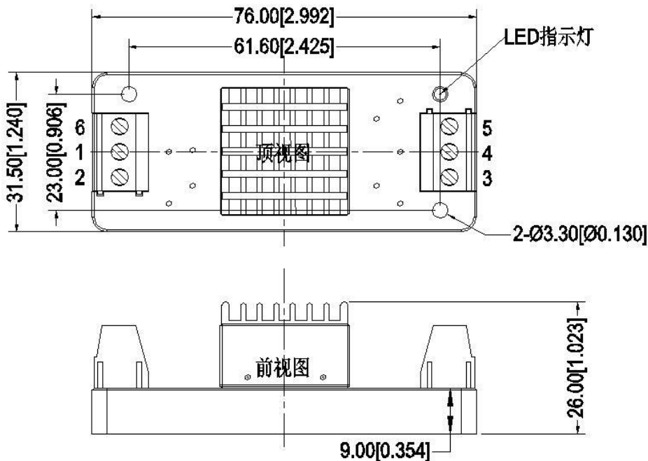
引脚定义
