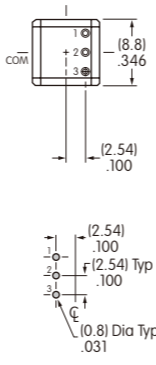
交替式
