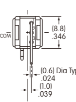
单极
