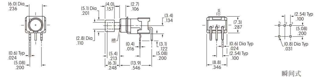
瞬间式
